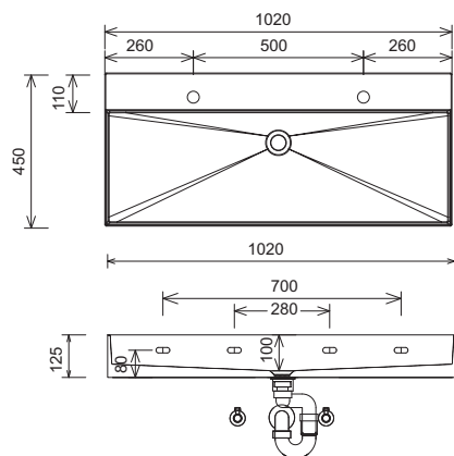
Squared 1020 Dvojité umyvadlo
