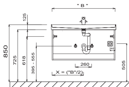
Umyvadlo Squared Skříňka pod umyvadlo s úchytem nebo bez úchyty
