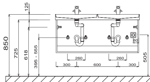
Dvojité umyvadlo Squared Skříňka pod umyvadlo s úchytem nebo bez úchyty
