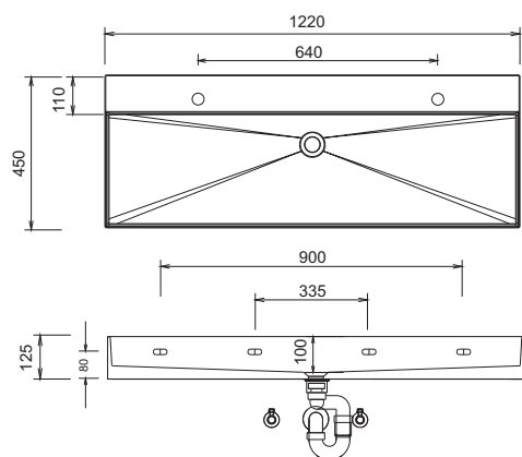
Squared 1220 Dvojité umyvadlo
