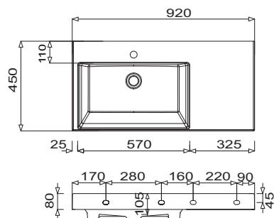
Q!flat 920 - police vpravo
